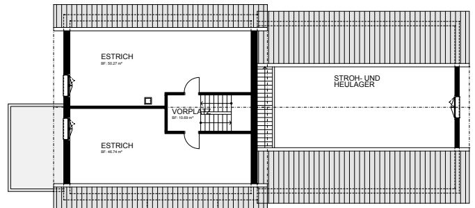
DACHGESCHOSS
