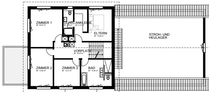
OBERGESCHOSS
